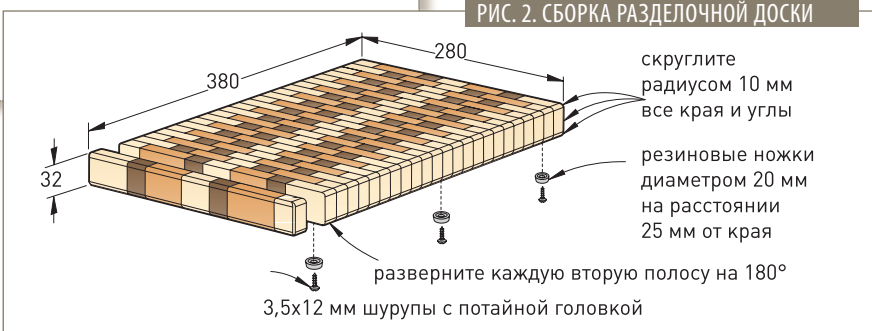
РИС. 2. СБОРКА РАЗДЕЛОЧНОЙ ДОСКИ
