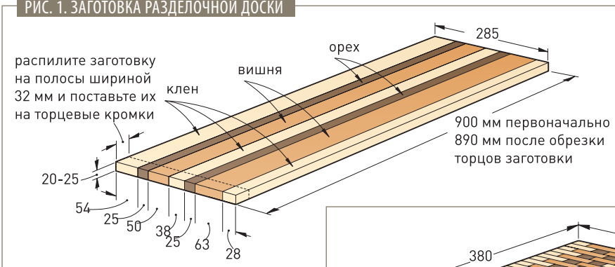
РИС. 1. ЗАГОТОВКА РАЗДЕЛОЧНОЙ ДОСКИ
